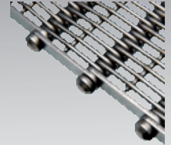
Typ 800 Drahtösengliedergurt
